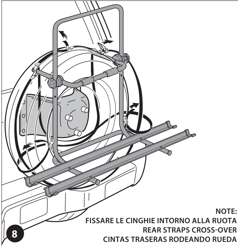
RUOTA A DESTRA SPARE WHEEL RIGHT RUEDA A LA DERECHA
